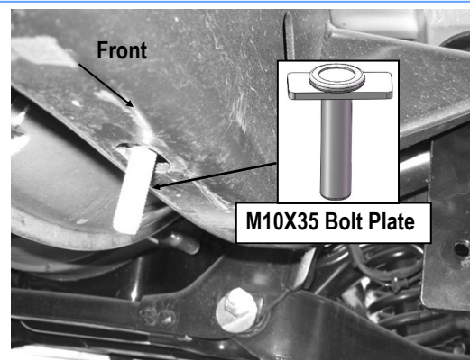
(Fig 5) Insert (1) M10X35 Bolt Plate
